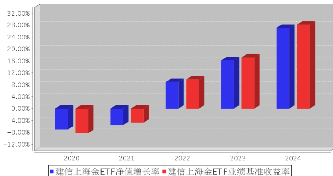
建信上海金ETF基金每年净值增长率与同期业绩比较基准收益率的对比图
