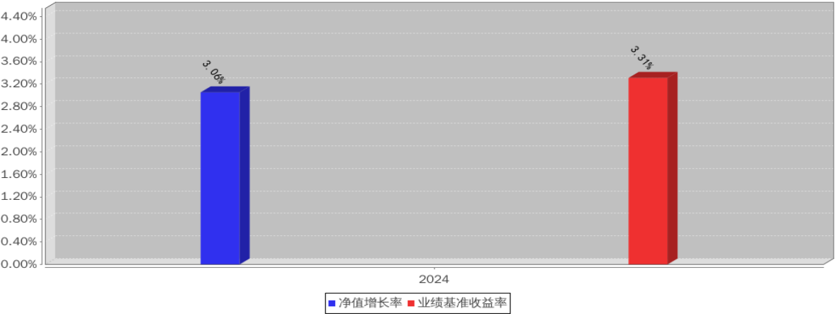
万家年年恒荣D基金每年净值增长率与同期业绩比较基准收益率的对比图（2024年12月31日）
