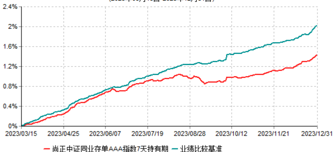
尚正中证同业存单AAA指数7天持有期证券投资基金累计净值增长率与业绩比较基准收益率历史走势对比图 (2023年03月15日-2023年12月31日)
