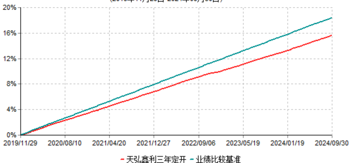
天弘鑫利三年定期开放债券型证券投资基金累计净值增长率与业绩比较基准收益率历史走势对比图 (2019年11月29日-2024年09月30日)
