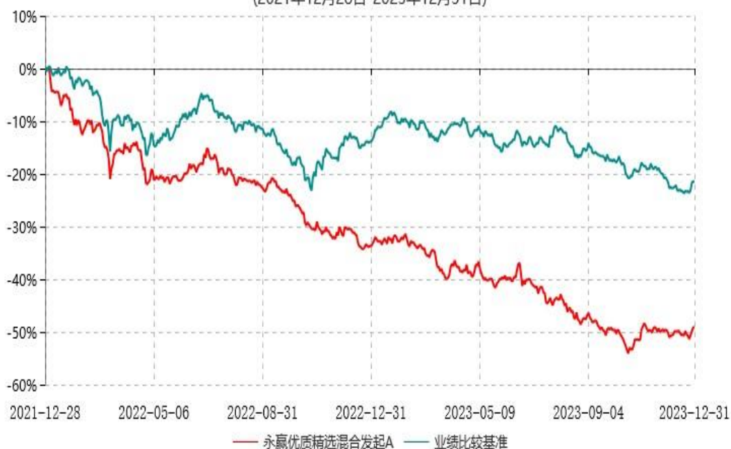
永赢优质精选混合发起A累计净值增长率与业绩比较基准收益率历史走势对比图
