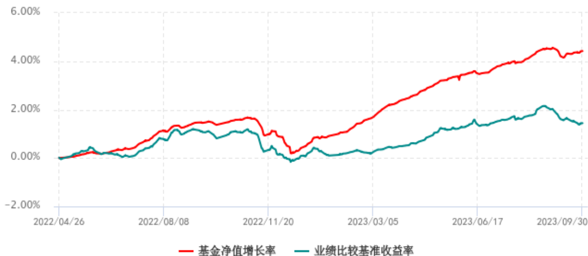
基金份额累计净值增长率与同期业绩比较基准收益率历史走势对比图 (2022年04月26日-2023年09月30日)
